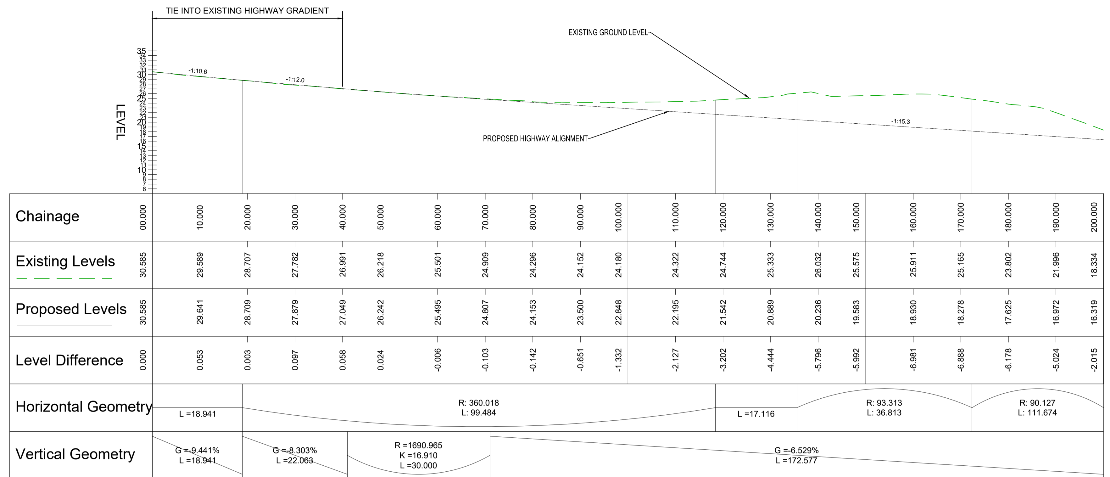
ROAD1 (CH.0-200) - LONGSECTION HORIZ 1:500, VERT 1:500. DATUM: 5.000m
