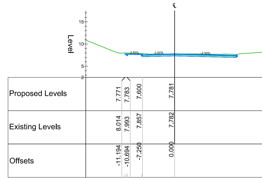
Chainage 420.000
