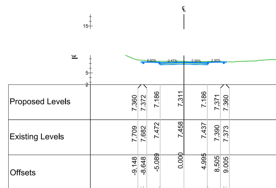
Chainage 400.000
