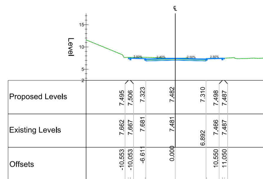
Chainage 410.000
