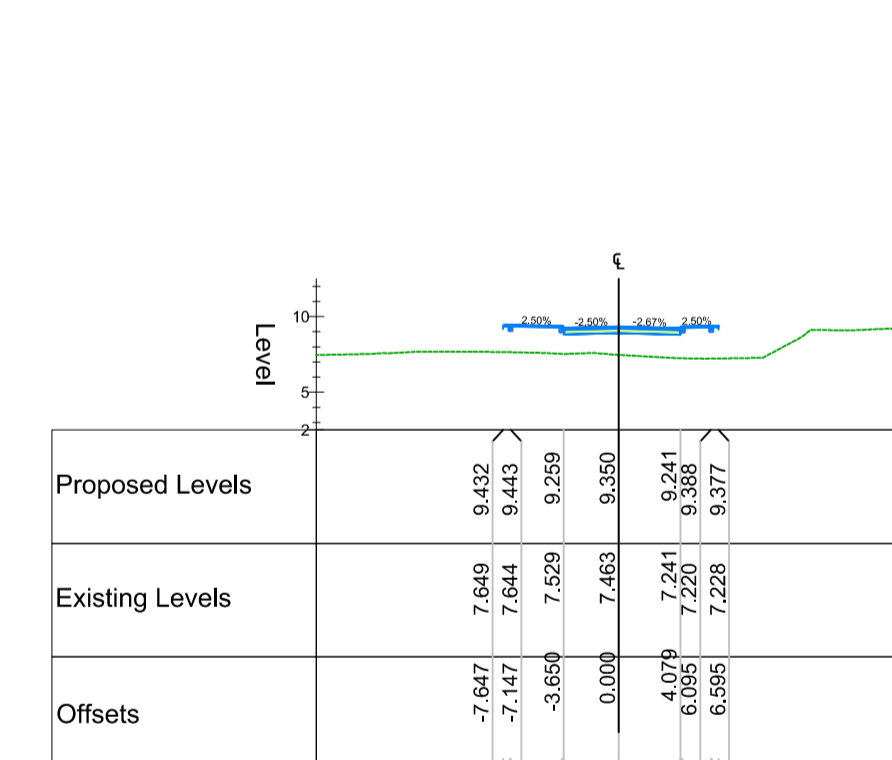
Chainage 370.000
