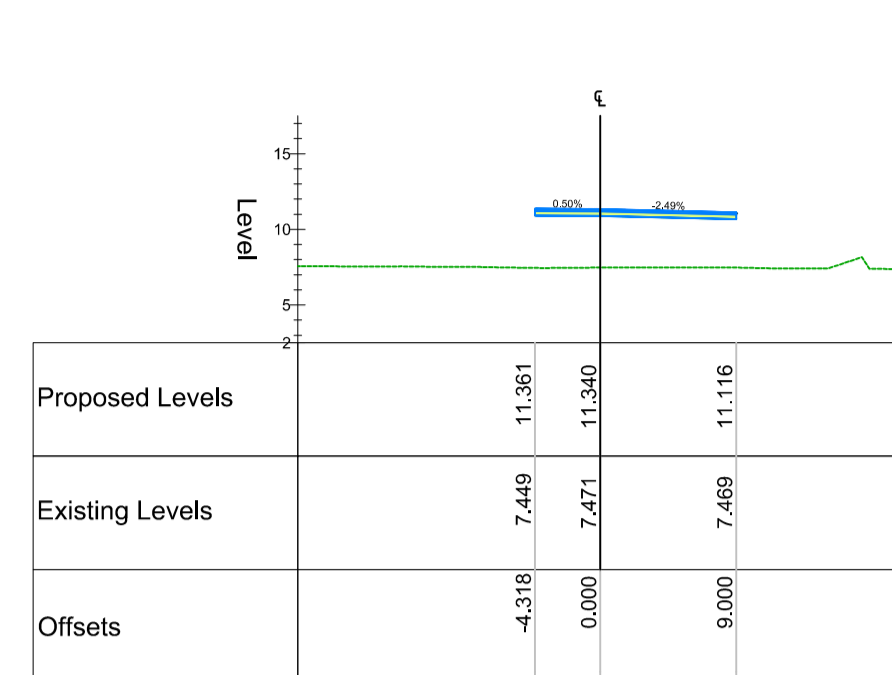
Chainage 310.000
