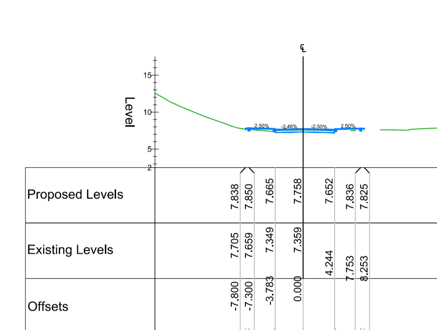
Chainage 390.000
