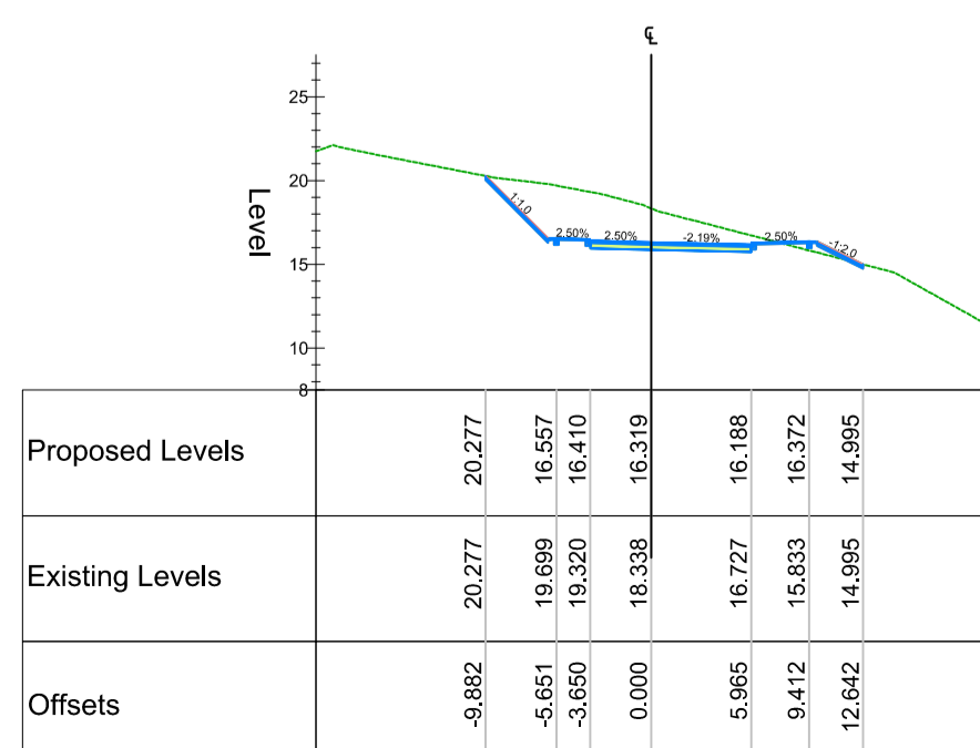
Chainage 200.000
