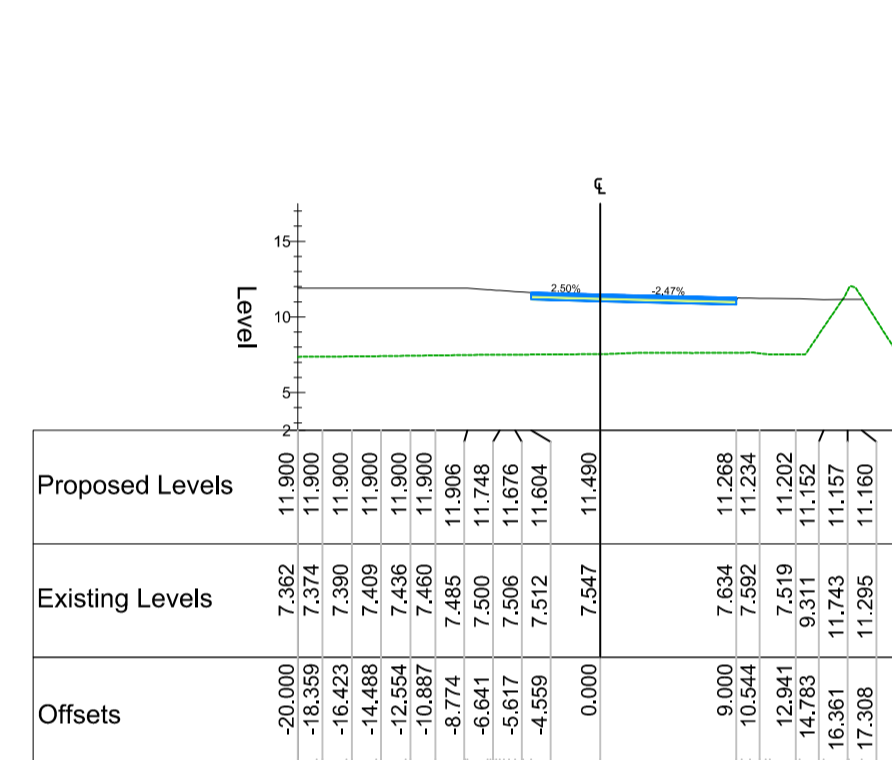
Chainage 300.000
