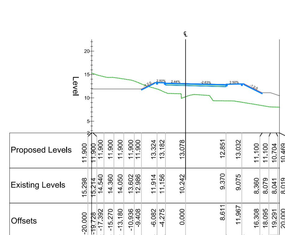
Chainage 250.000
