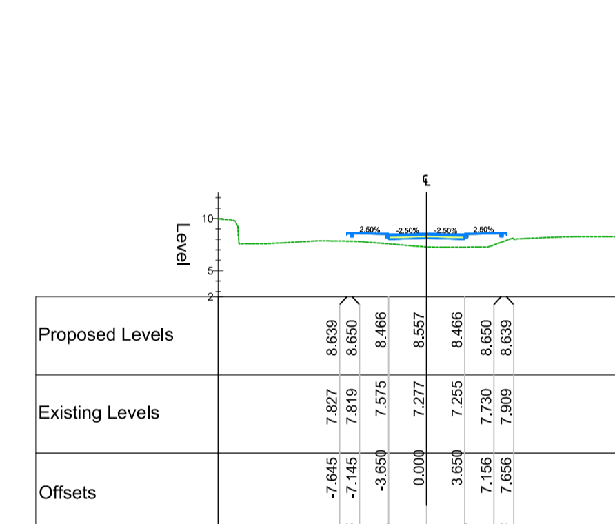
Chainage 380.000
