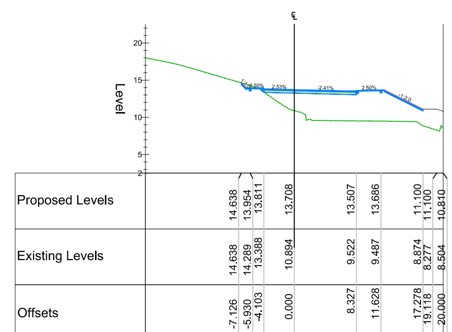
Chainage 240.000
