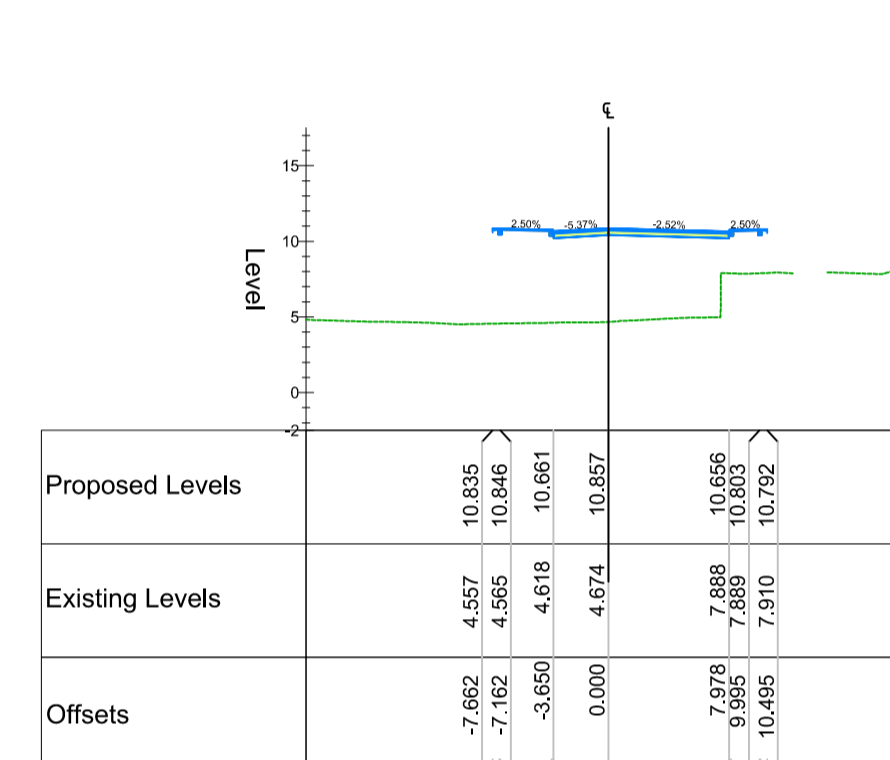
Chainage 340.000
