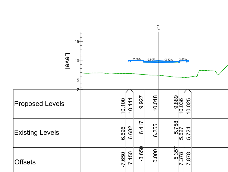
Chainage 360.000
