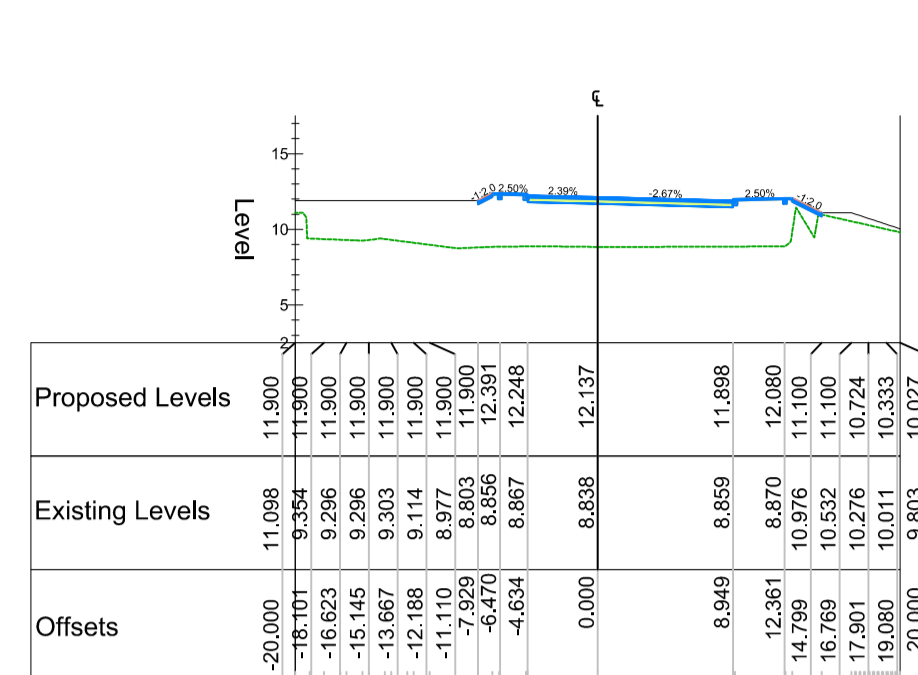
Chainage 270.000
