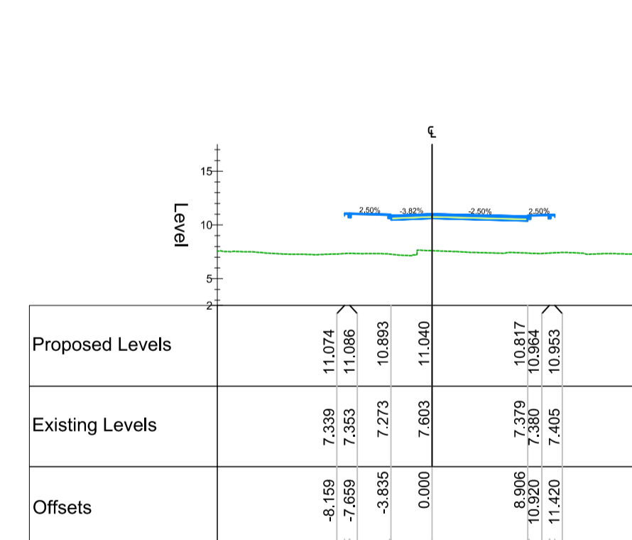
Chainage 330.000
