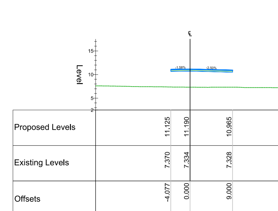
Chainage 320.000
