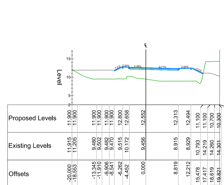
Chainage 260.000
