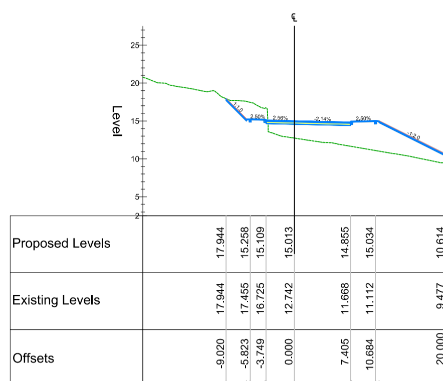
Chainage 220.000
