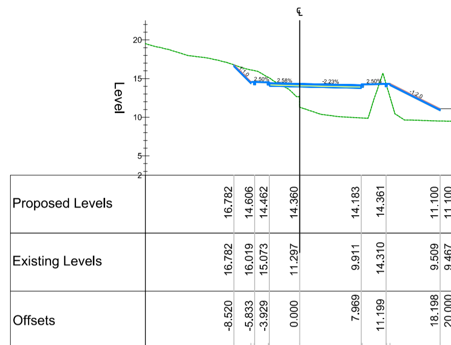
Chainage 230.000
