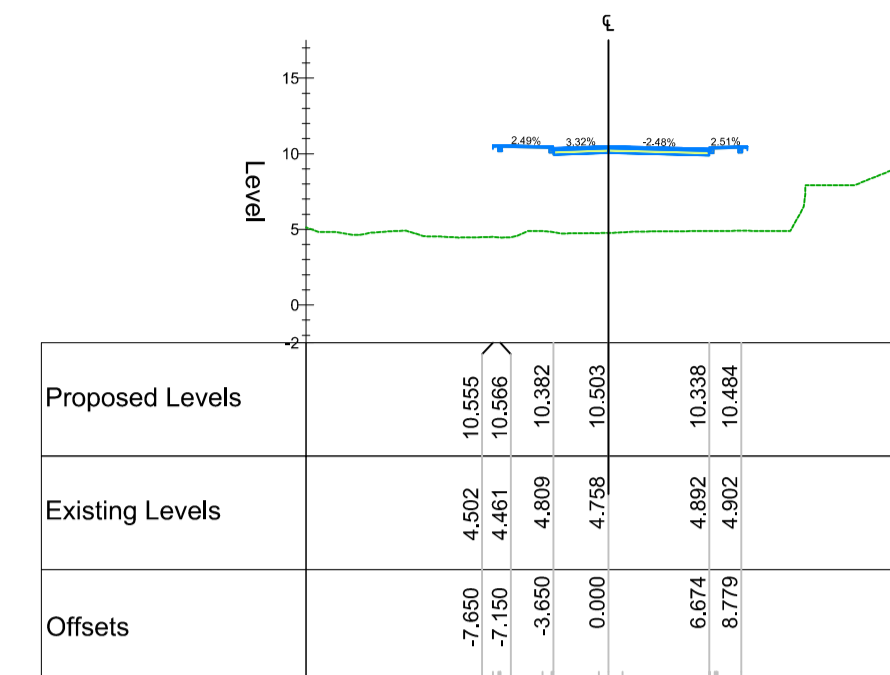
Chainage 350.000
