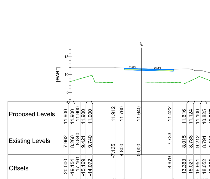
Chainage 290.000
