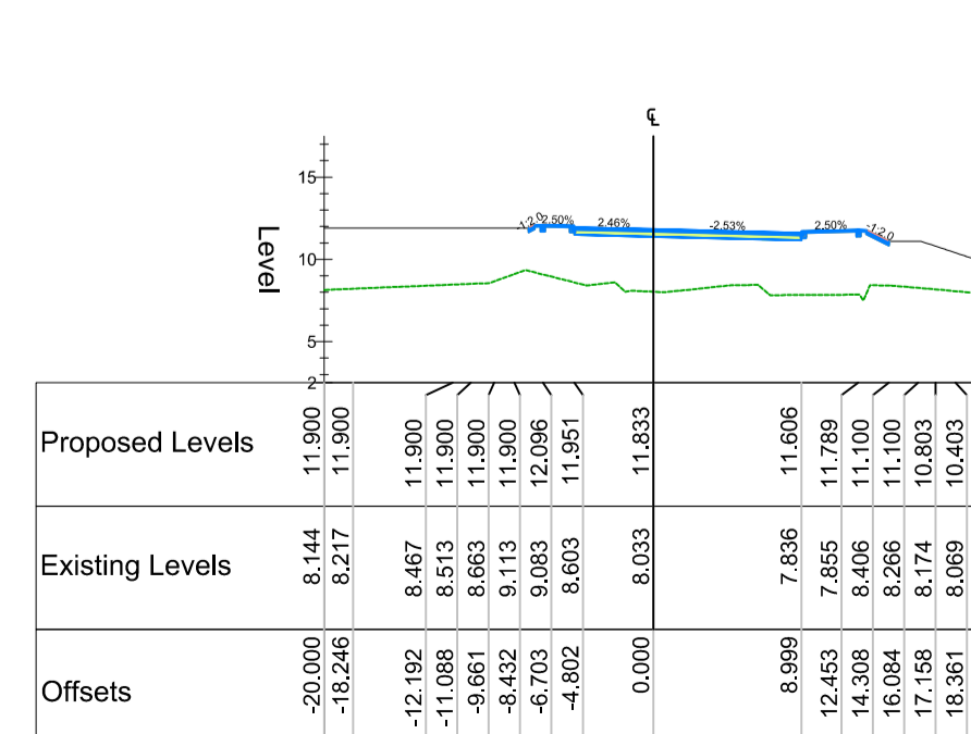
Chainage 280.000
