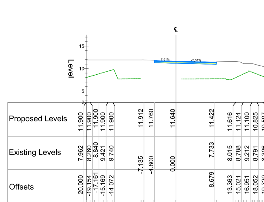
Chainage 290.000
