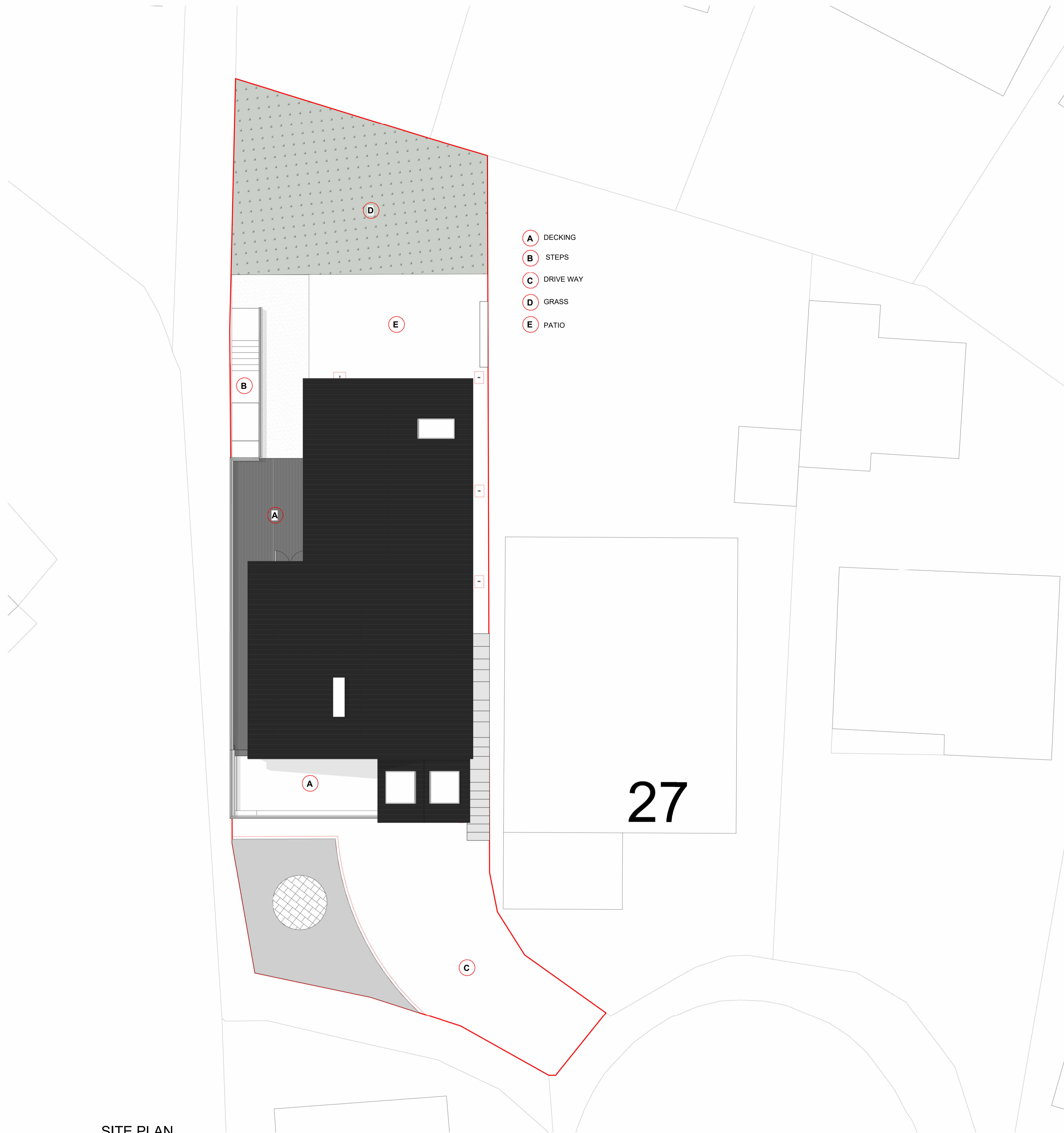
SITE PLAN 1 : 100
