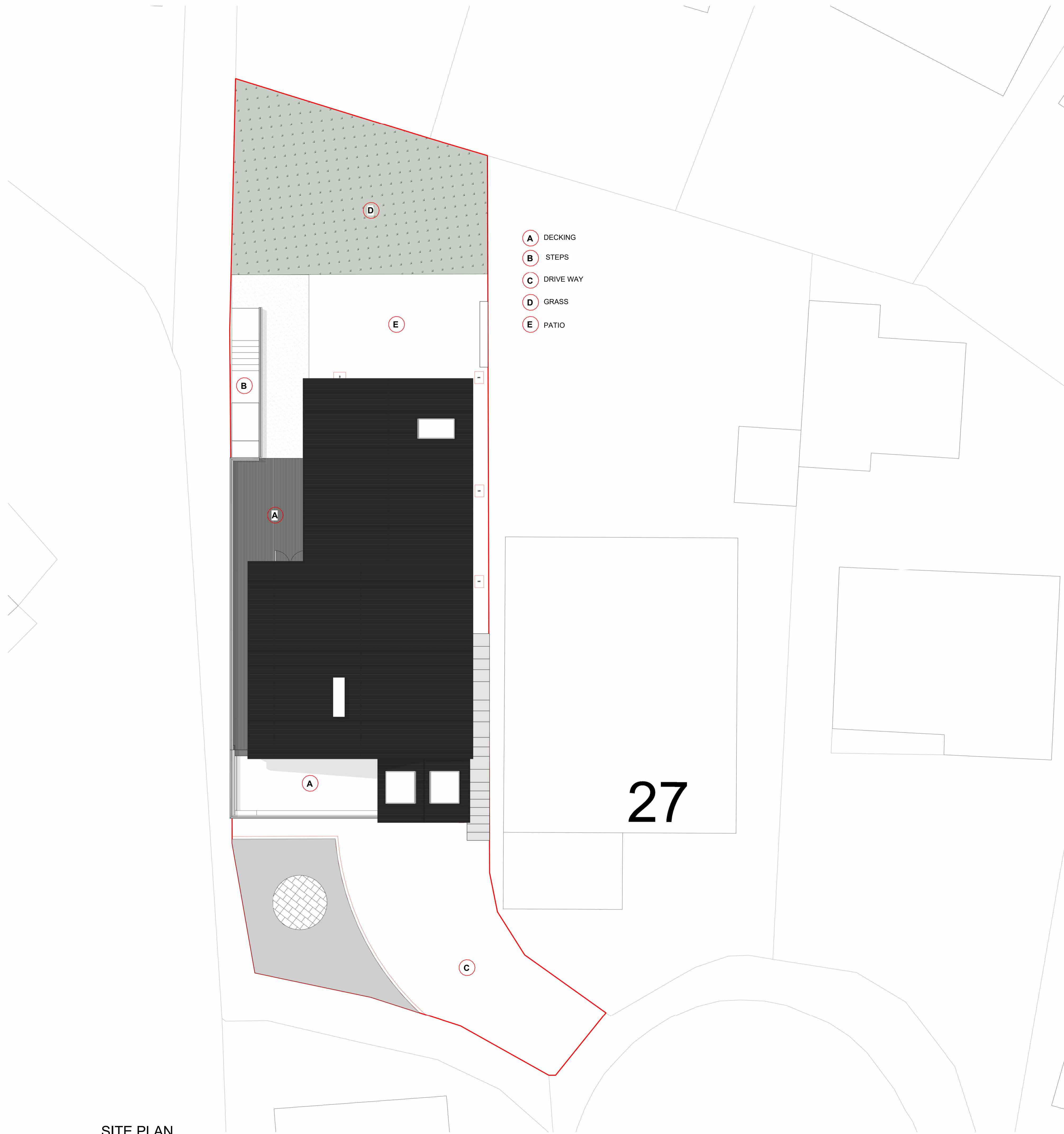
SITE PLAN 1 : 100
