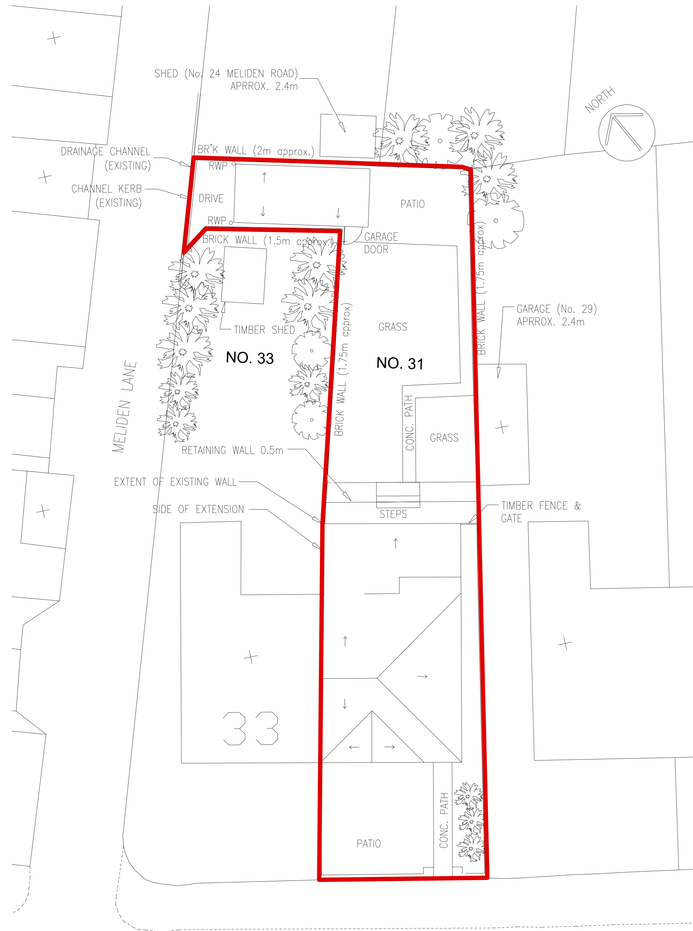
EXISTING SITE PLAN 1:100
